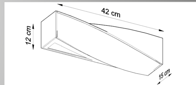
SZKIC TECHNICZNY Z WYMIARAMI
